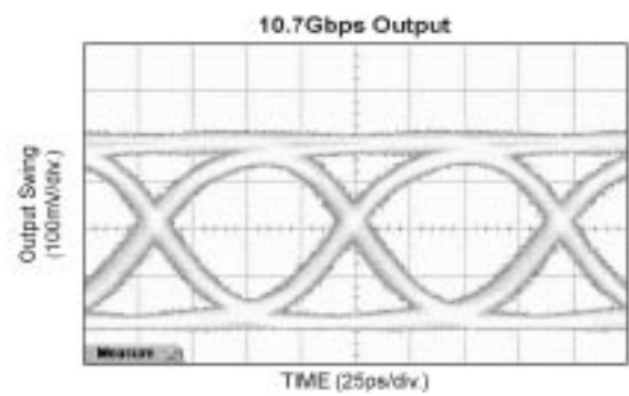
( 2^{23}-1 PRBS Pattern)
